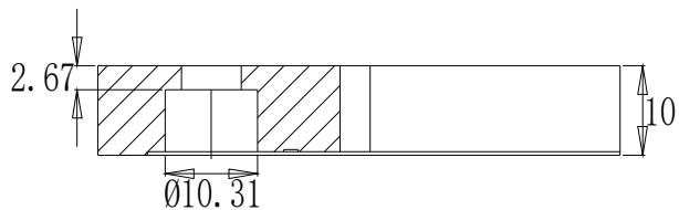
截面 A-A
